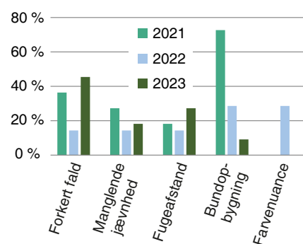
Figur 43: Brolægning og hårde belægninger
