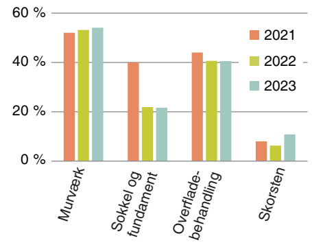
Figur 41: Udførelsesmæssige problemer ved murerarbejde
