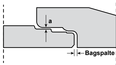
Udformning af spids- og mufteende i beton (EURO)
