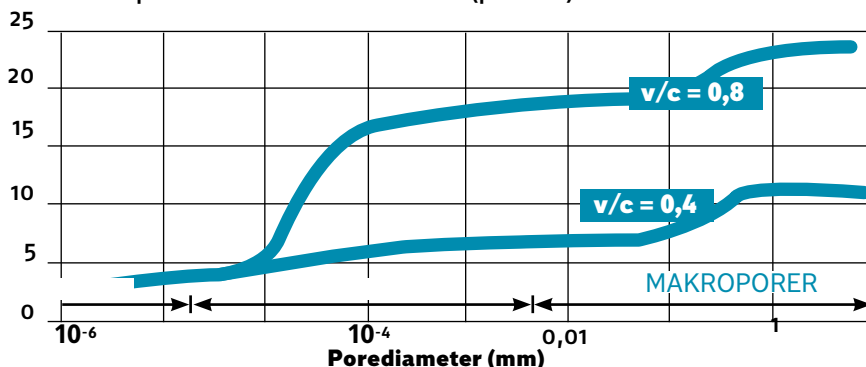
Kumuleret porevolumen/betenvolumen (procent)
