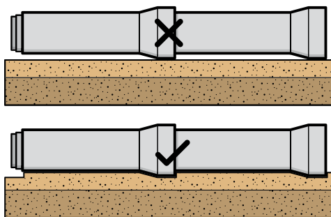
Muffehuller sikrer, at det er rørkroppen, der bærer vægten
