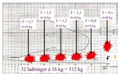
Plan for sprængning
