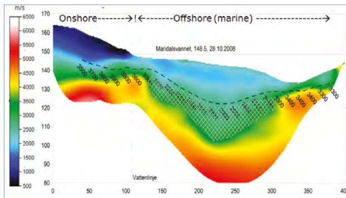
Typisk resultat af refraktionsseismisk undersøgelse. Skalaen til venstre viser transmissionshastigheder i undergrunden. Maridalssvannet, Oslo 2008. Rambøll
