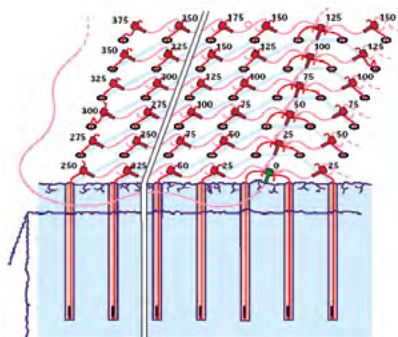
Principskitse for opladning og sprængning med millisekundsinkelse
