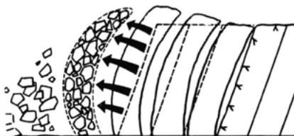
Skitsen viser princippet for udnyttelse af millisekundsinkelse mellem sprængladningerne i bjergsprængning
